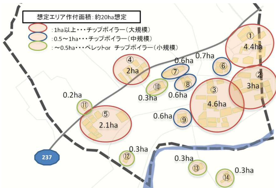
図 4.2-1 荷菜地区農業ハウスの木質バイオマス活用の例
